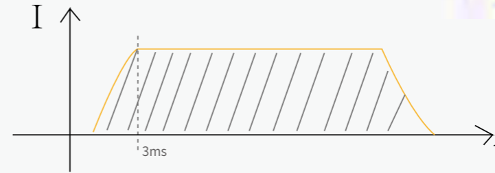
中频直流放电曲线 Medium Frequency DC Discharge Curve
